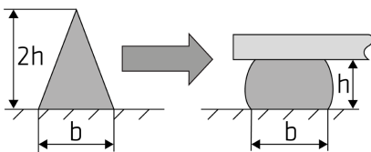
Figur 1: Anbefalet trekantskonfiguration
