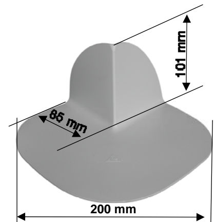
S-hjørne PVC 90° A
