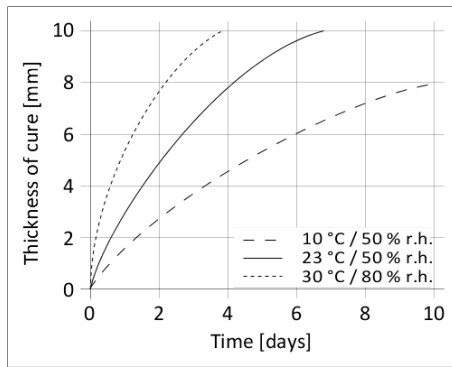
Diagram 1: Hærdningshastighed SikaTack® Panel-50
