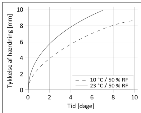
Diagram 1: Hærdehastighed for Sikaflex®-290 DC PRO
