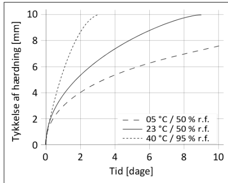
Diagram 1: Hærdhastighed Sikasil® WS-200
