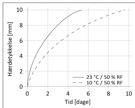
Diagram 1: Hærdehastighed for Sikaflex®-298 FC
