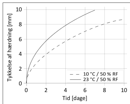
Diagram 1: Hærdehastighed for Sikaflex®-290 DC PRO
