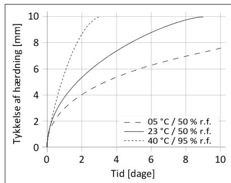
Diagram 1: Hærdhastighed Sikasil® WS-200
