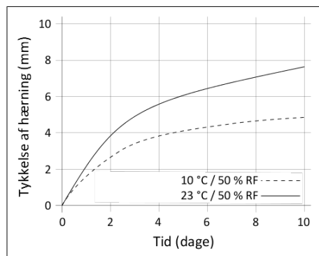
Diagram 1: Hærdhastighed for Sikaflex®-529 Evolution
