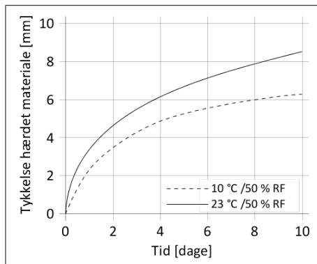
Diagram 1: Hærdningshastighed Sikaflex®-552 AT
